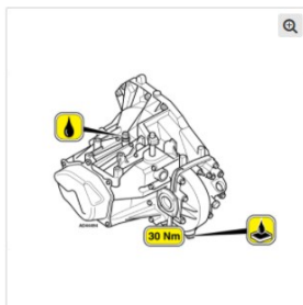
Механическая коробка переключения передач
