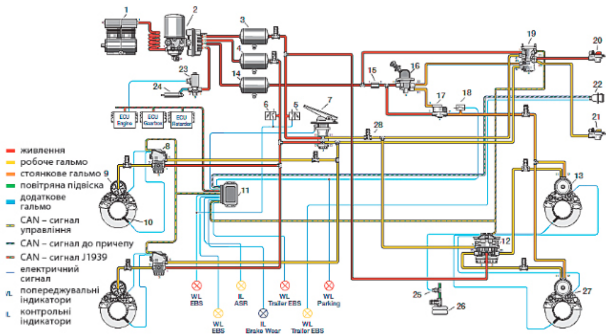
5. Схема автомобільної електропневматичної гальмівної системи (EBS) (джерело: Knorr-Bremse)
