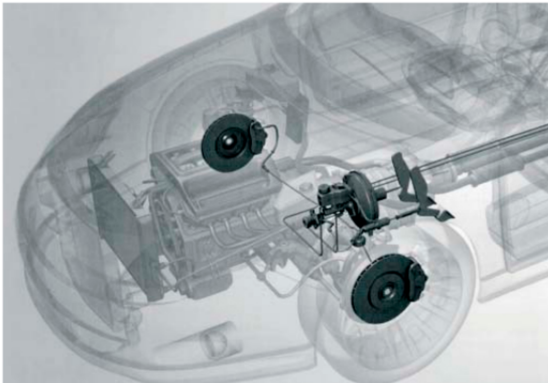
3. Схема двоконтурної гальмівної системи з гідравлічним управлінням, яка застосовується в легковому автомобілі (джерело: FTE automotive)
