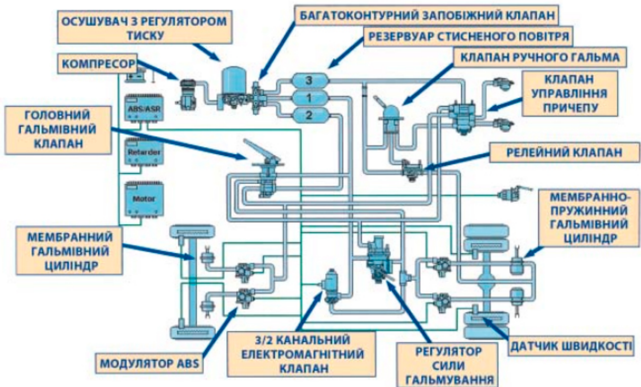
4. Схема пневматичної гальмівної системи вантажного автомобіля (джерело: Wabco)
