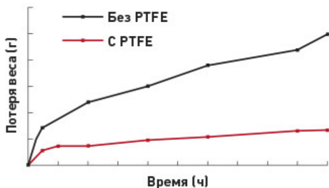
Рис.1. Ремни с покрытием из PTFE демонстрируют значительно меньшую потерю материала, то есть более устойчивы к истиранию.
